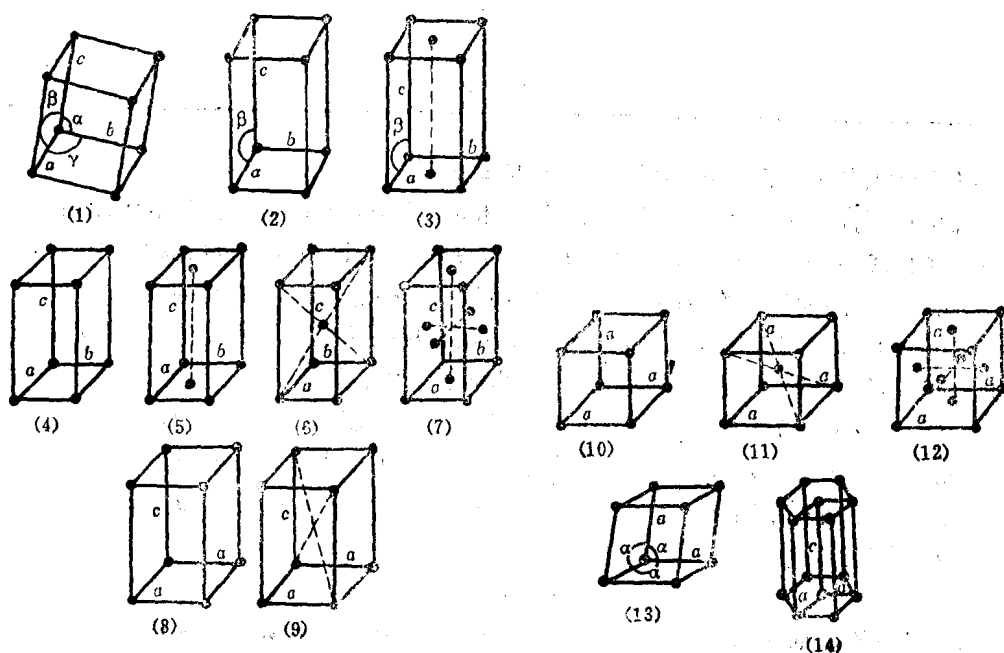
图1-1 十四种布喇菲格子
