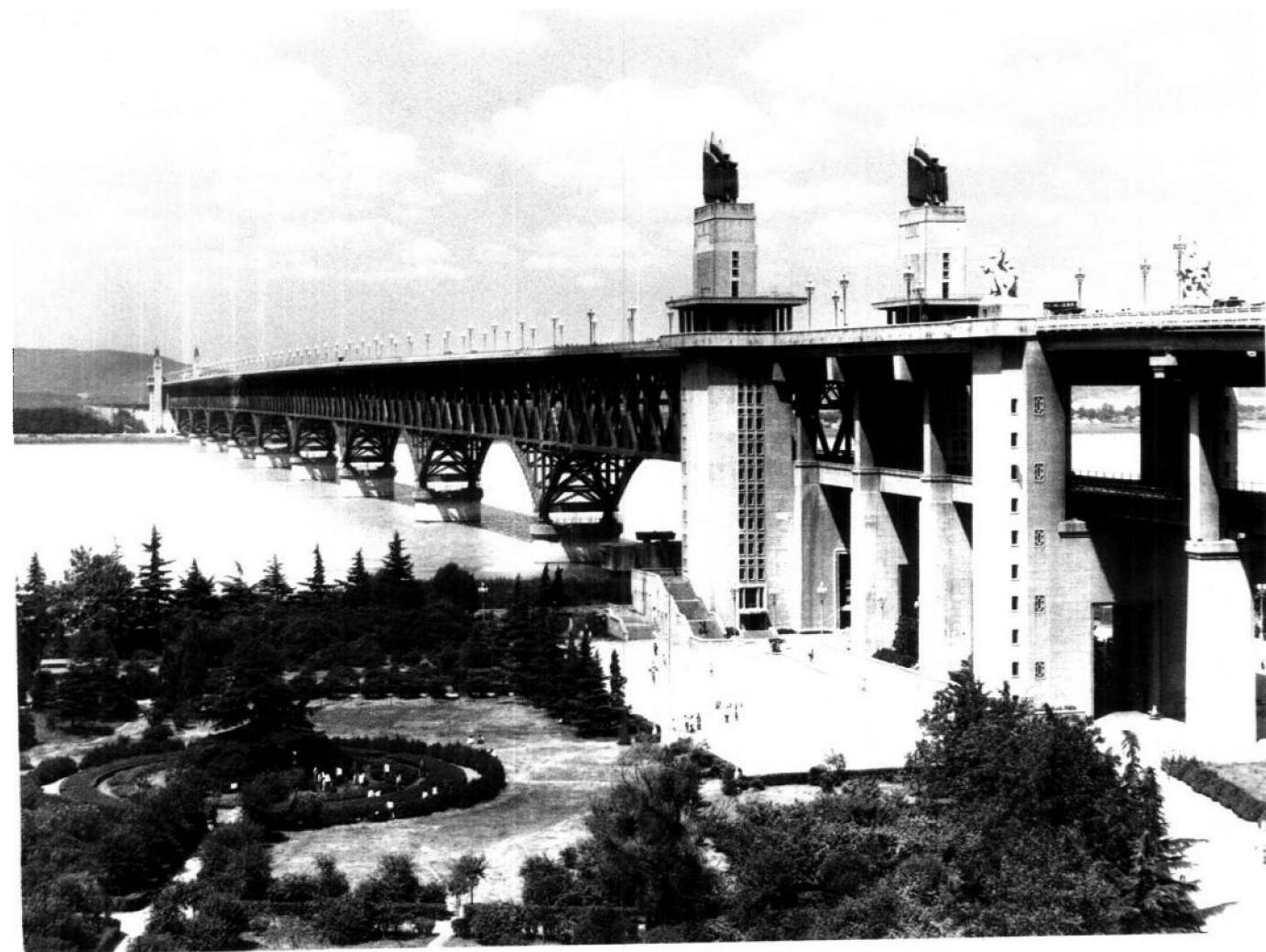
南京长江大桥桥头堡
