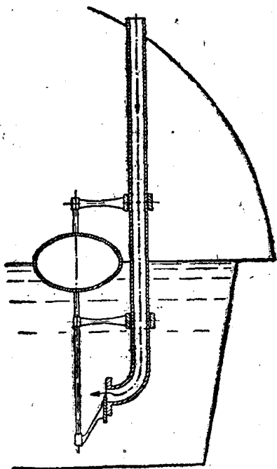
圖 1. 保爾祖諾夫的給水調節器簡圖。
