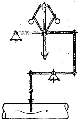
圖 2. 瓦特的轉數調節器簡圖。
