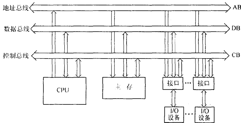
图 1.6 典型的标准总线结构
