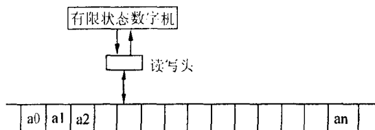
图 1.2 Turing 机器
