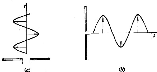
图1.7 水平和垂直极化波 (a)水平极化波；(b)垂直极化波。
