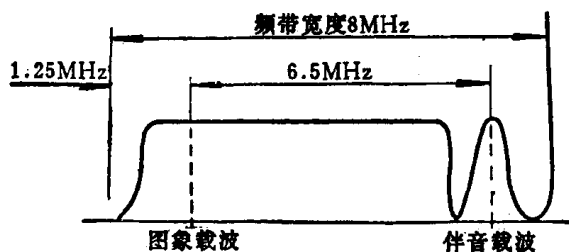
图 1.2 电视的频道宽度
