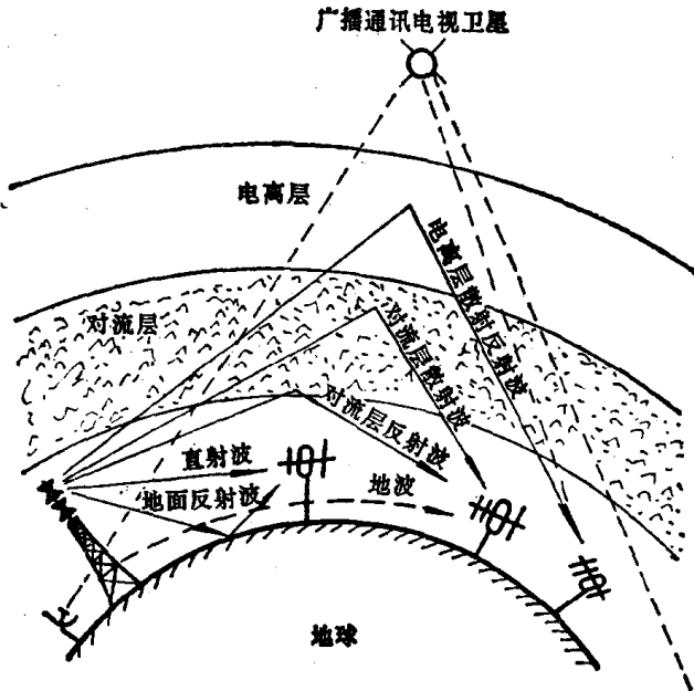
图1.3 电视广播信号的传播途径
