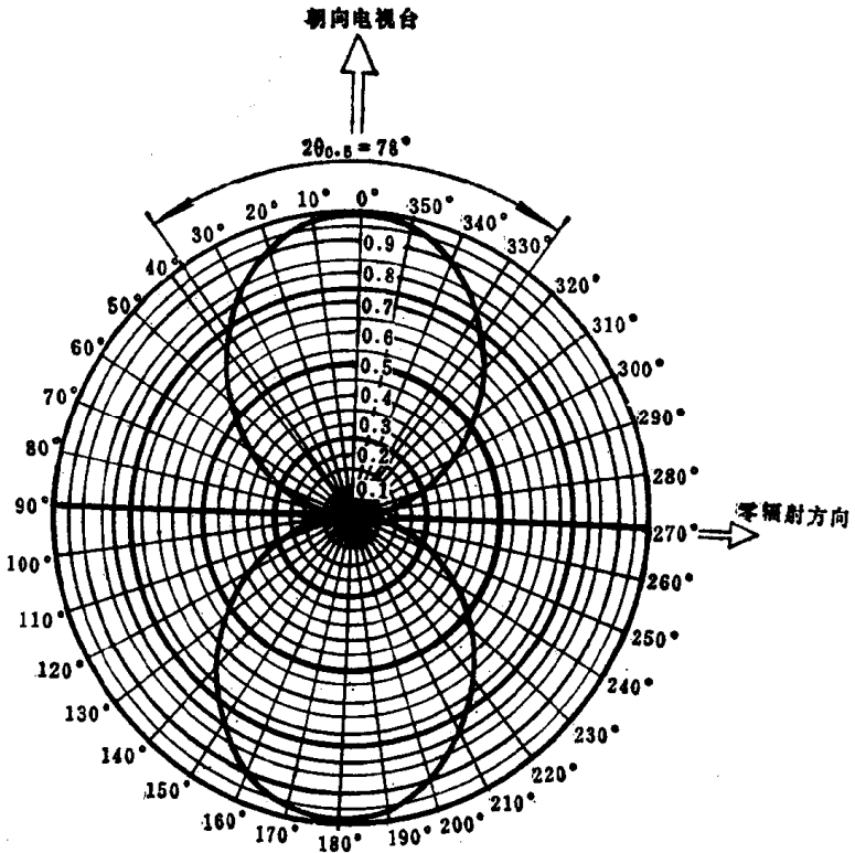
图1.5 半波振子归一化水平面场强方向图
