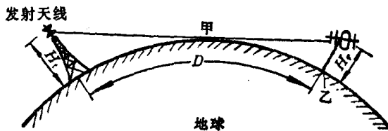
图1.4 直视距离与地球曲率的关系
