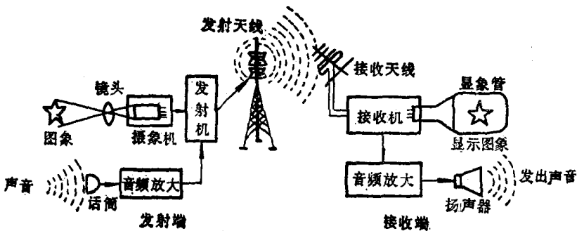
图1.1 电视信号的发射与接收
