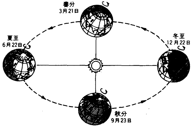
图 2.7 地球的公转
