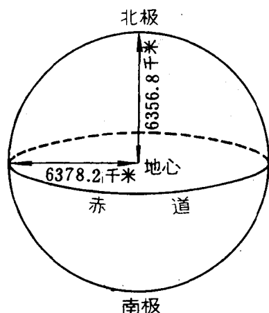
图 2.1 地球的大小
