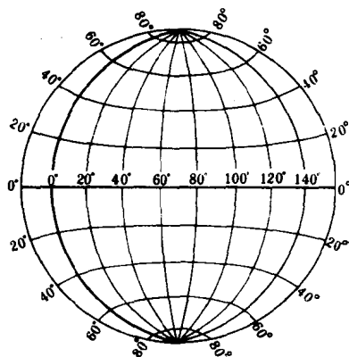
图 2.4 经纬网
