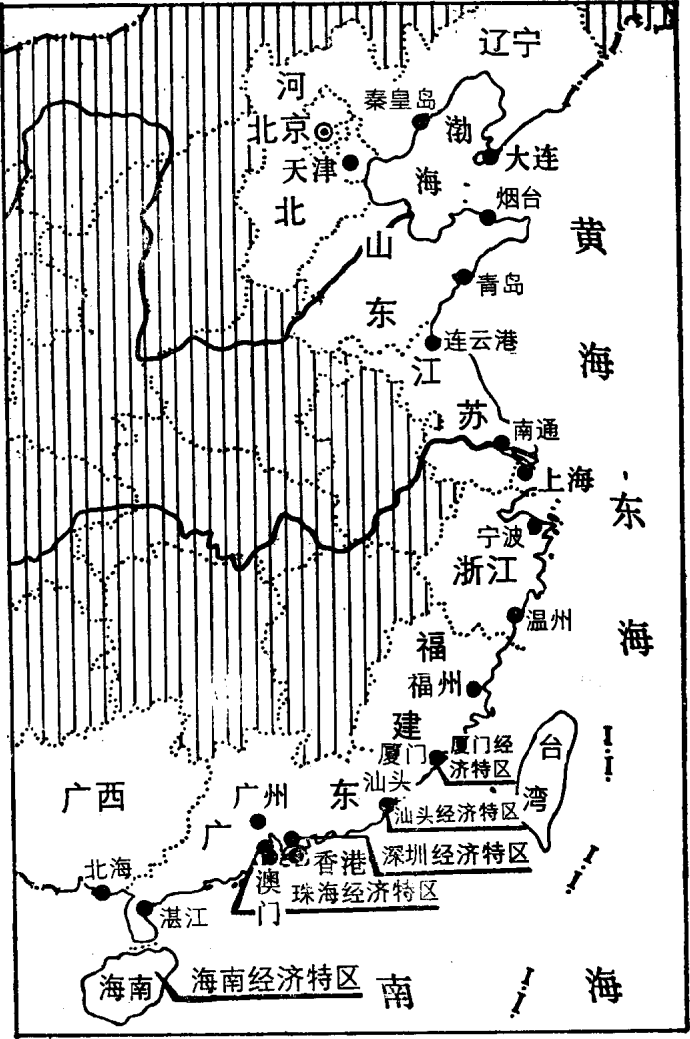
中国沿海经济特区、开放港口城市示意图
