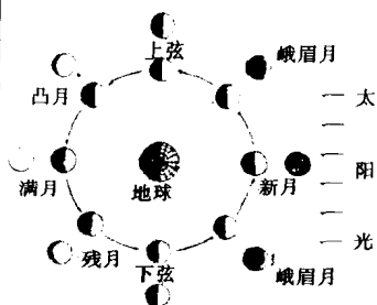
月相变化图
