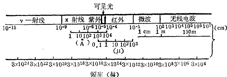
图（1—2）电磁波谱
