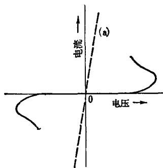
图 3.3 Ge 片与 Ge 片接触时的电流-电压特性
