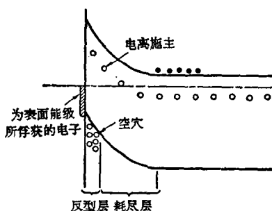
图 3.5 有表面能级时的能带图
