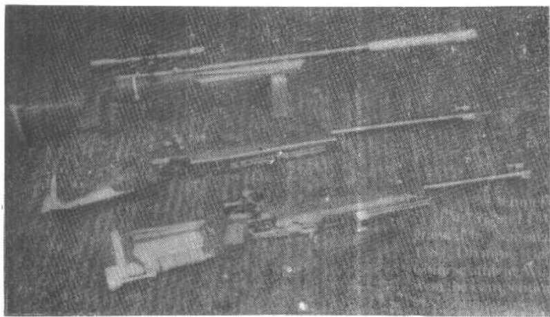
解放后建设机床厂生产的小口径比赛用步枪。
