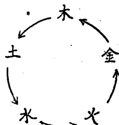
图2. 五行相尅
