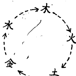
图1. 五行相生
