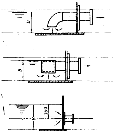
图1-7 出油管和“死藏”高度 B
