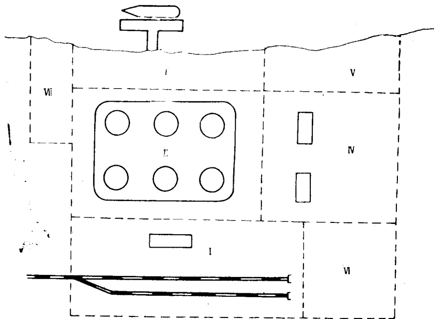
图1-5 油库分区示意图
