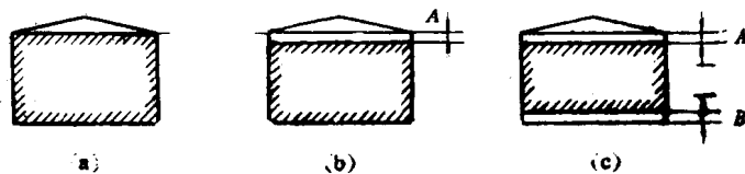
图1-6 油罐容量的使用情况
