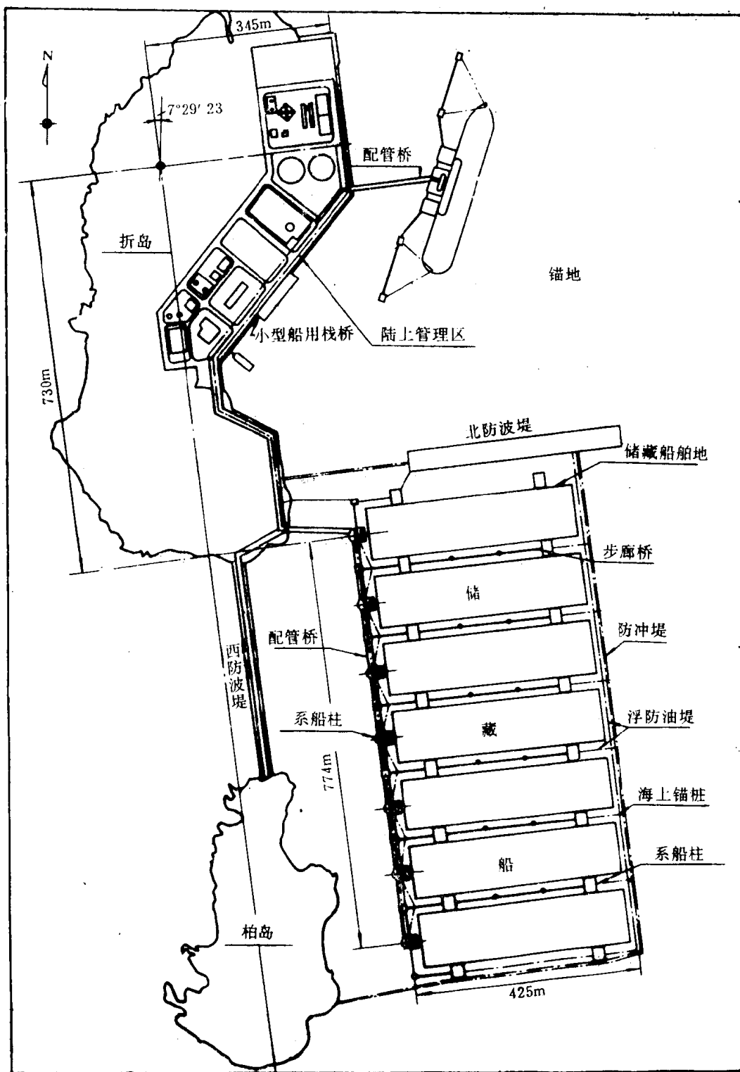
图1-3 飘浮式海上油库概貌
