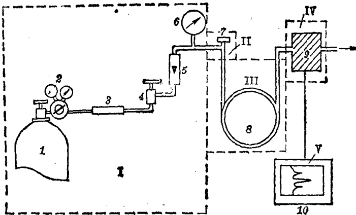
图2-1 气相色谱流程图
