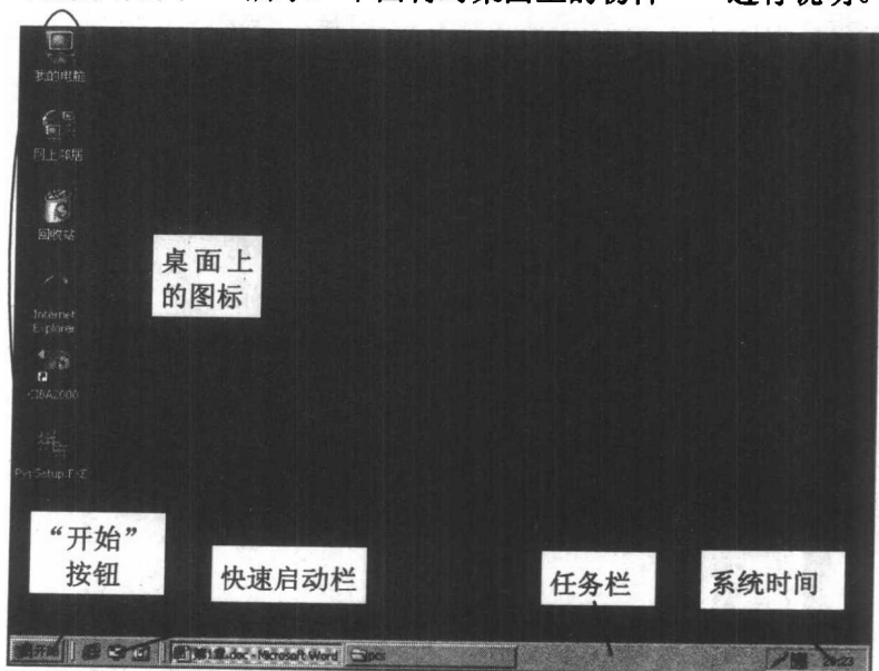
图 1-1 Windows 2000 的桌面
