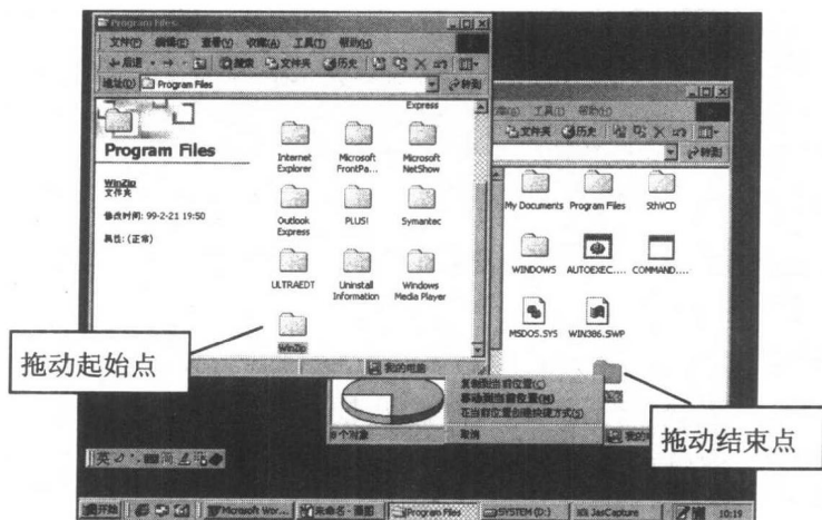
图 1-17 鼠标的拖动
