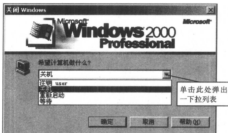
图 1-12 退出 Windows
