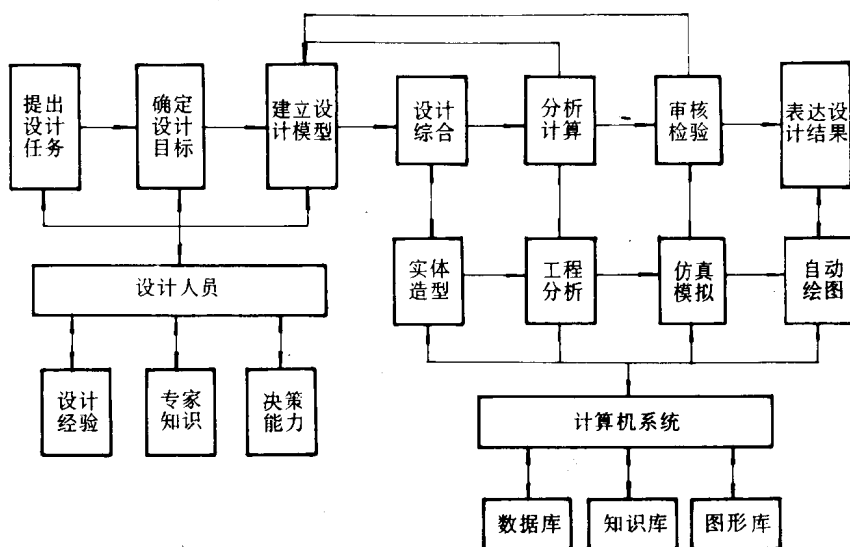
图 1-1 计算机辅助设计系统示意图
