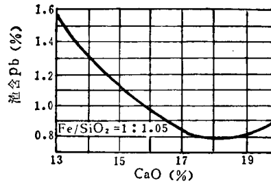
图 4—1—3 炉渣中氧化钙量对渣含铅的影响
