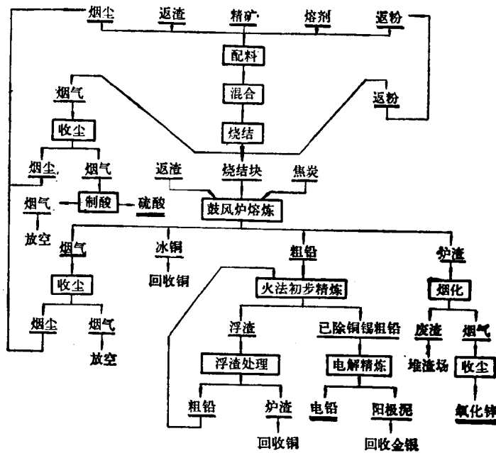
图 4—1—1 鼓风炉炼铅工艺流程图
