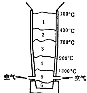
图 4—1—2 鼓风炉内区域划分示意图
