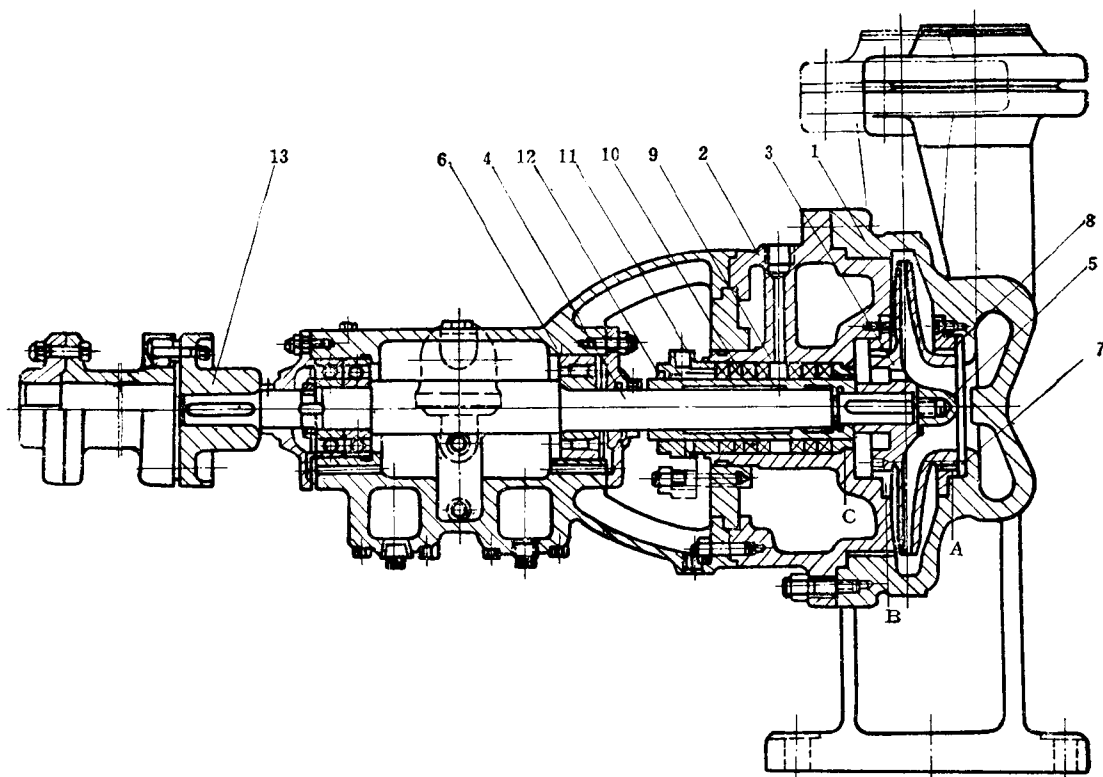
图 1—2 单级单吸悬臂式Y型油泵结构图 (10)
