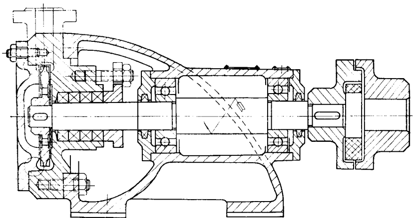
图 1—8 W型旋涡泵结构图
