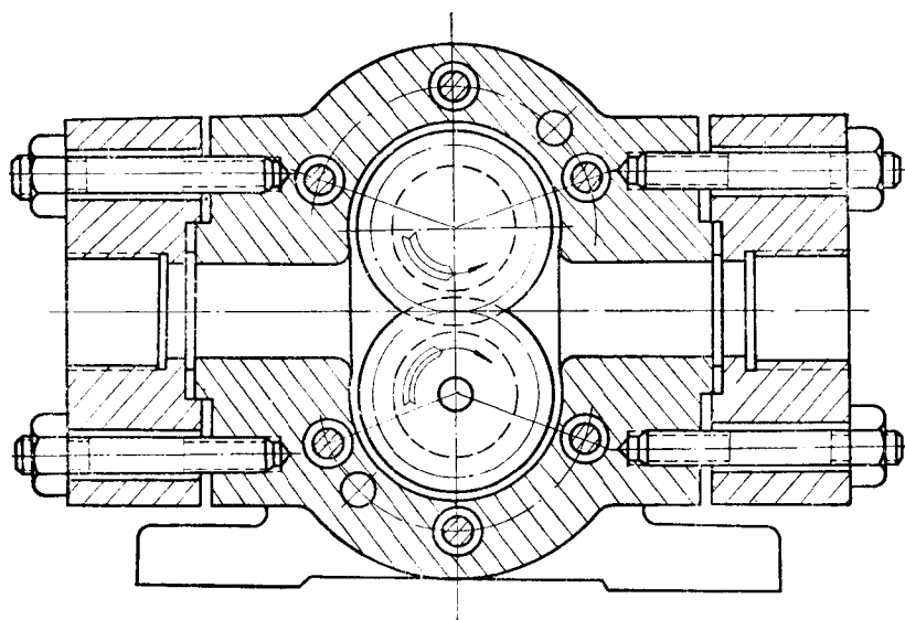
图 1—9 Ch型齿轮泵结构图
