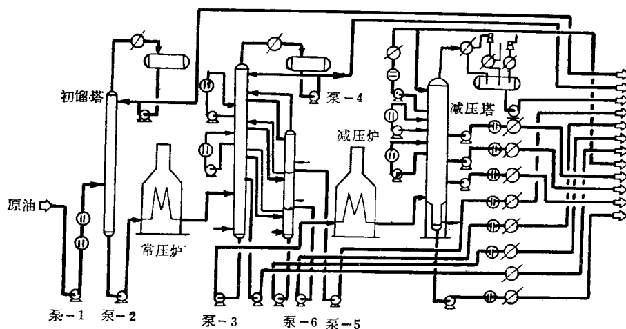
图 1—1 常减压蒸馏装置工艺流程示意图
