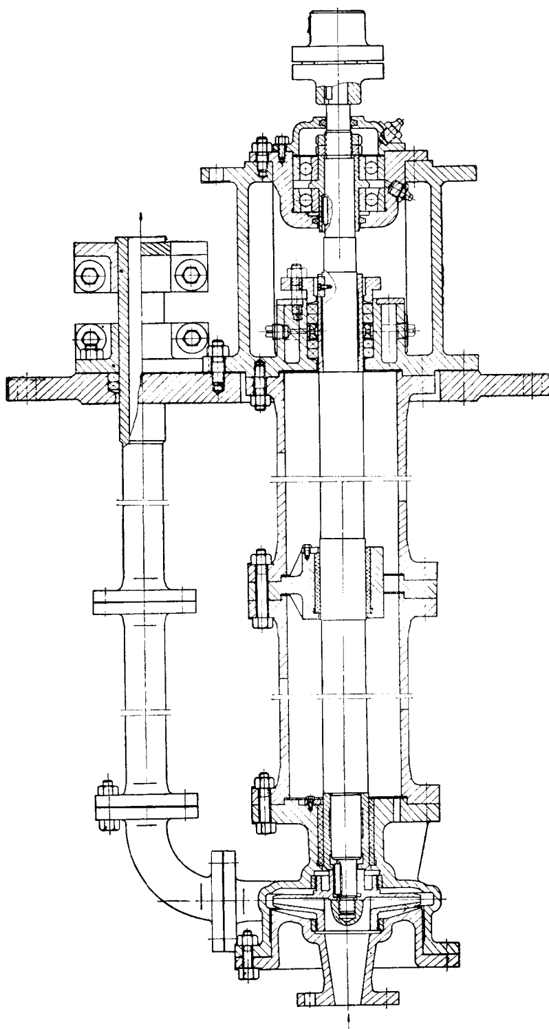
图 1-7 FY型液下耐腐蚀离心泵结构图
