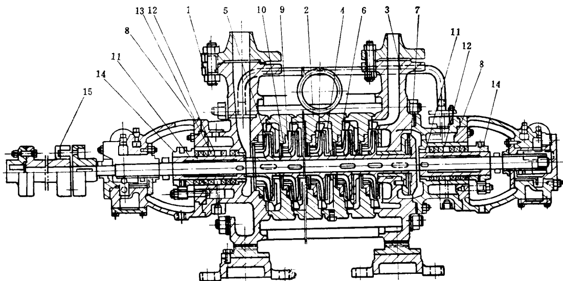
图 1—3 多级节段式 Y 型油泵结构图 (10)
