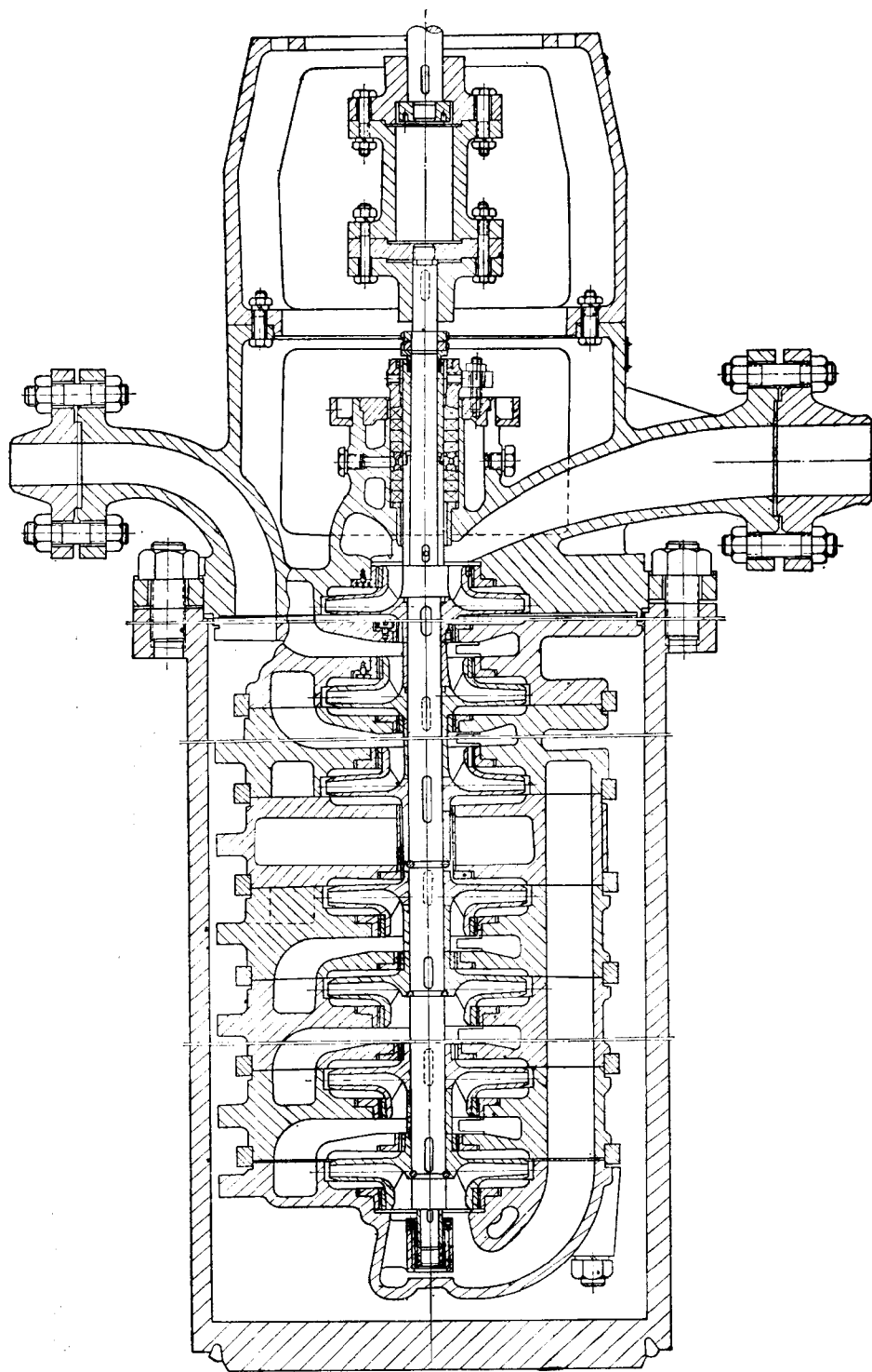
图 1—5 3YT-5×24型筒式离心油泵结构图
