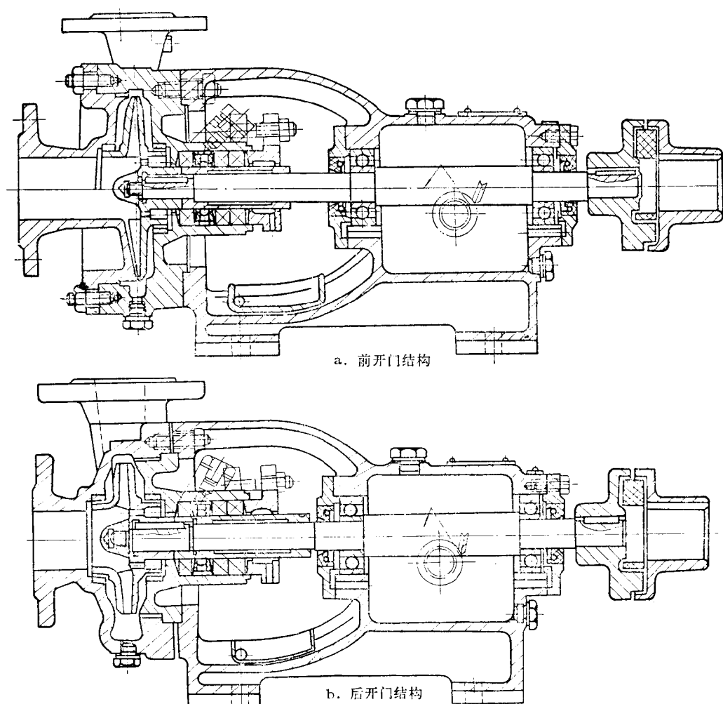
图 1—6 F型耐腐蚀泵结构图
