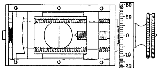
圖 1-14 目鏡測微計。
