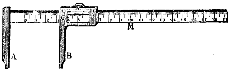
圖 1-5 游標測徑器。
