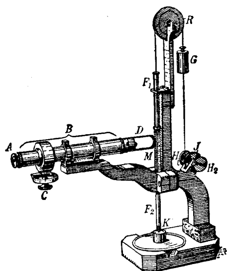
圖 1-13 蔡司測厚器。
