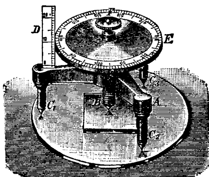
圖 1-11 球徑計。
