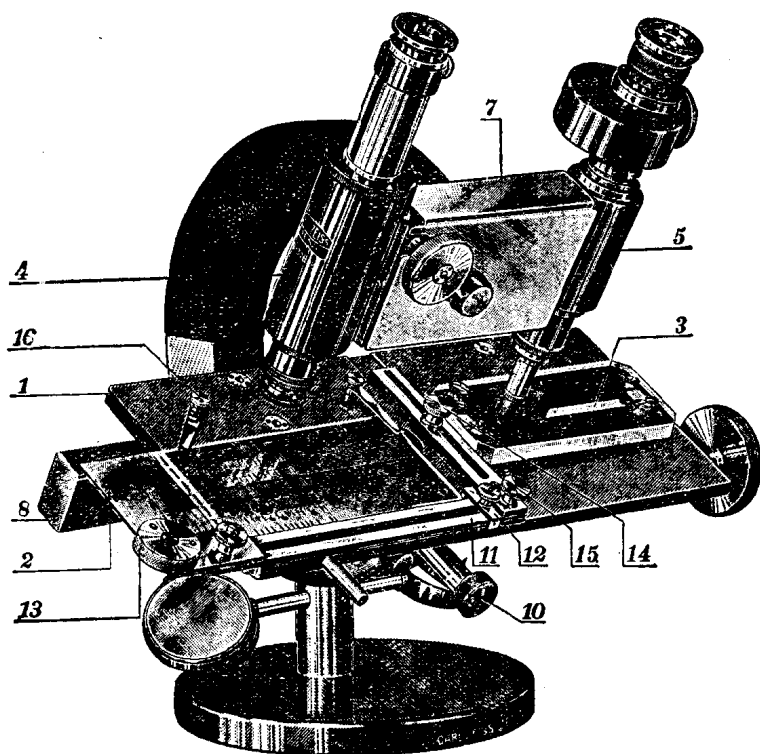
圖 1-8 阿俾比長儀。
