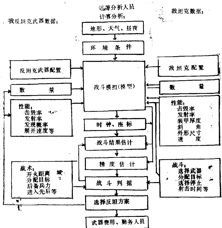
反坦克模型方框图
