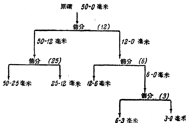
圖 3 聯合篩分作業流程圖 (括號內是篩孔尺寸)
