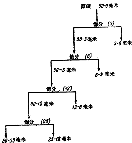
圖 2 依次獲得由細到粗級別的篩分作業流程圖 (括號內的是篩孔尺寸)
