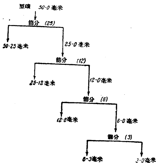
圖 1 依次獲得由粗到細級別的篩分作業流程圖 (括號內的是篩孔尺寸)
