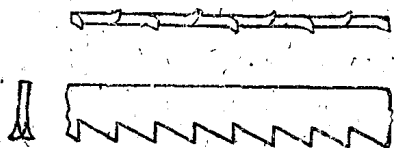
圖 2·5 縱鋸齒
