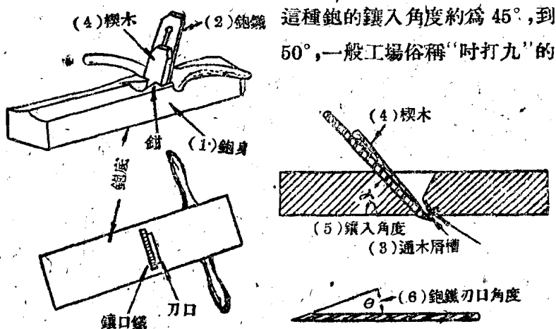
圖 2-10 平鉋
