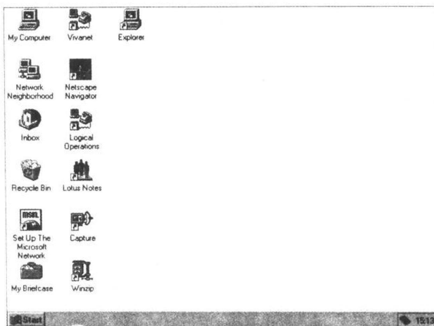
图 1-1 Windows95 桌面
