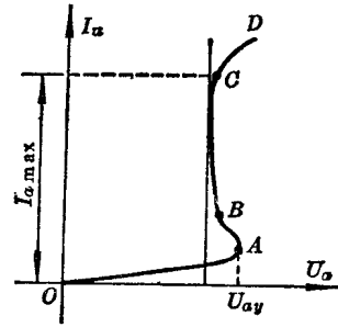
图1-2-3 充气二极管的伏安特性曲线
