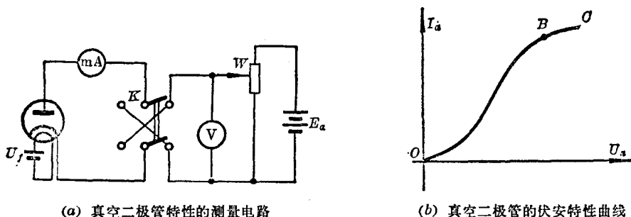
图 1-1-3 真空二极管特性的测量电路及其伏安特性曲线
