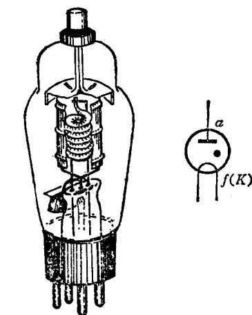
(a) 充气二极管的构造 (b) 充气二极管的符号 图 1-2-1 充气二极管的构造及其符号
