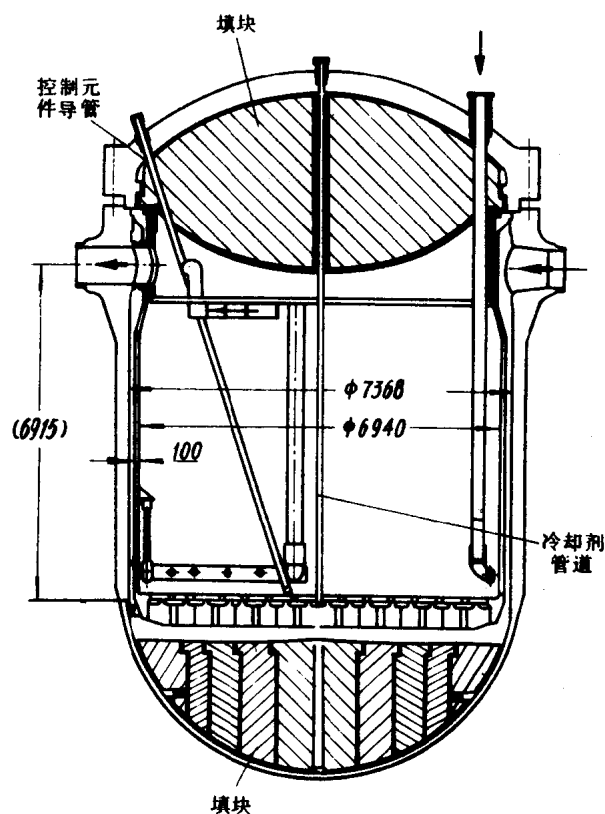
图 1-1 压力壳式重水反应堆示意图
