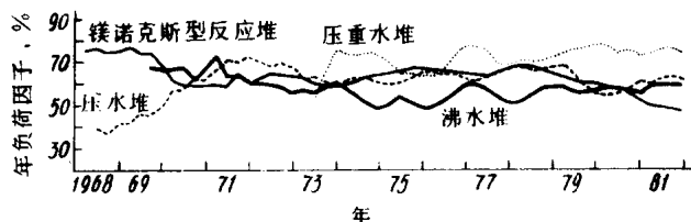
图 1-5 几种主要堆型的负荷因子
