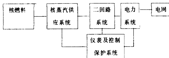
图 1-6 核电站主要组成部分
