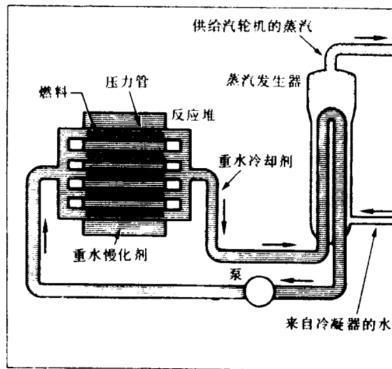
图 1-2 坎杜压重水反应堆示意图
