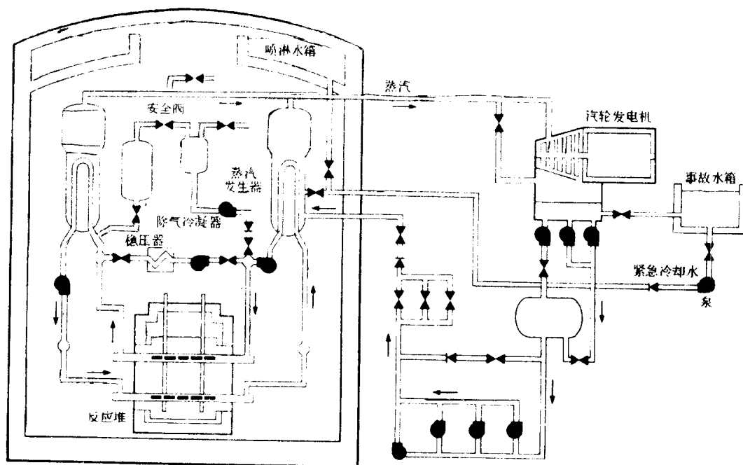
图 1-7 重水堆核电站工艺系统原理流程
