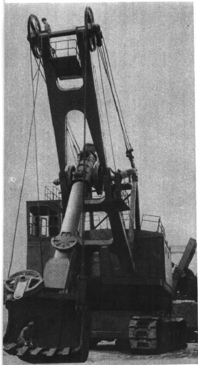
十立方米大型挖掘机。
