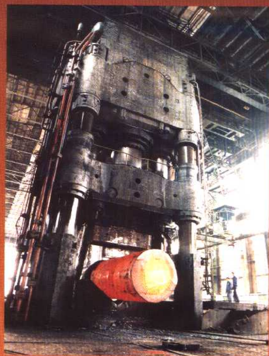
德阳第二重型机器厂拥有的万吨 水压机 二重 供稿
