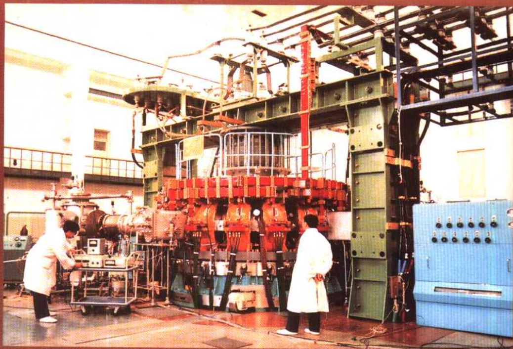
我国最大的受控核聚变实验装置——中国环流器一号
