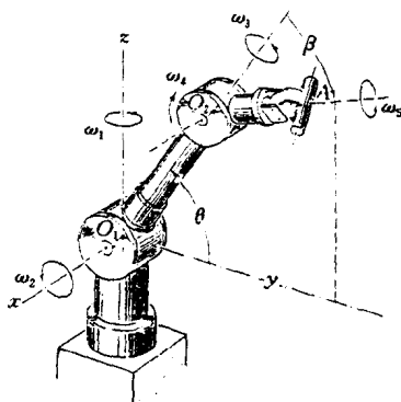
图 3 五自由度机械臂
