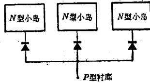
图2.5 被反向偏置PN结隔离的小岛模型
