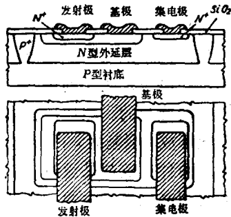
图2.3 用PN结隔离的集成晶体管
