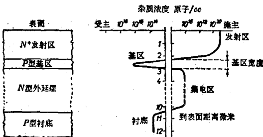
图2.4 NPN晶体管典型掺杂的纵剖面图
