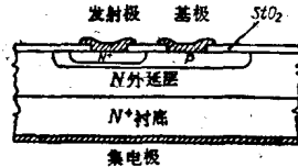
图2.1 硅外延平面晶体管的横截面
