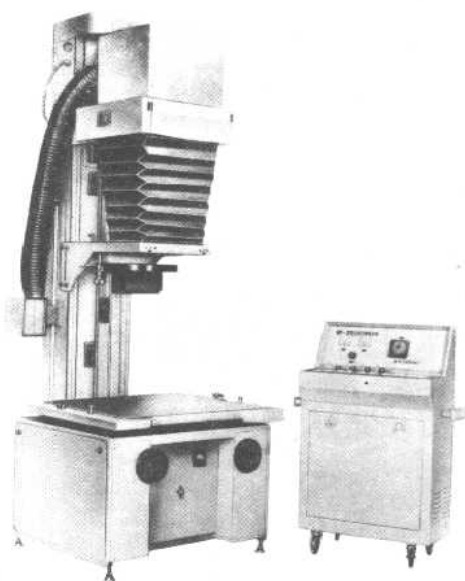
QFC 强光源 立式分色放大机
