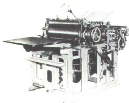
TZ401 四开停回转印刷机
