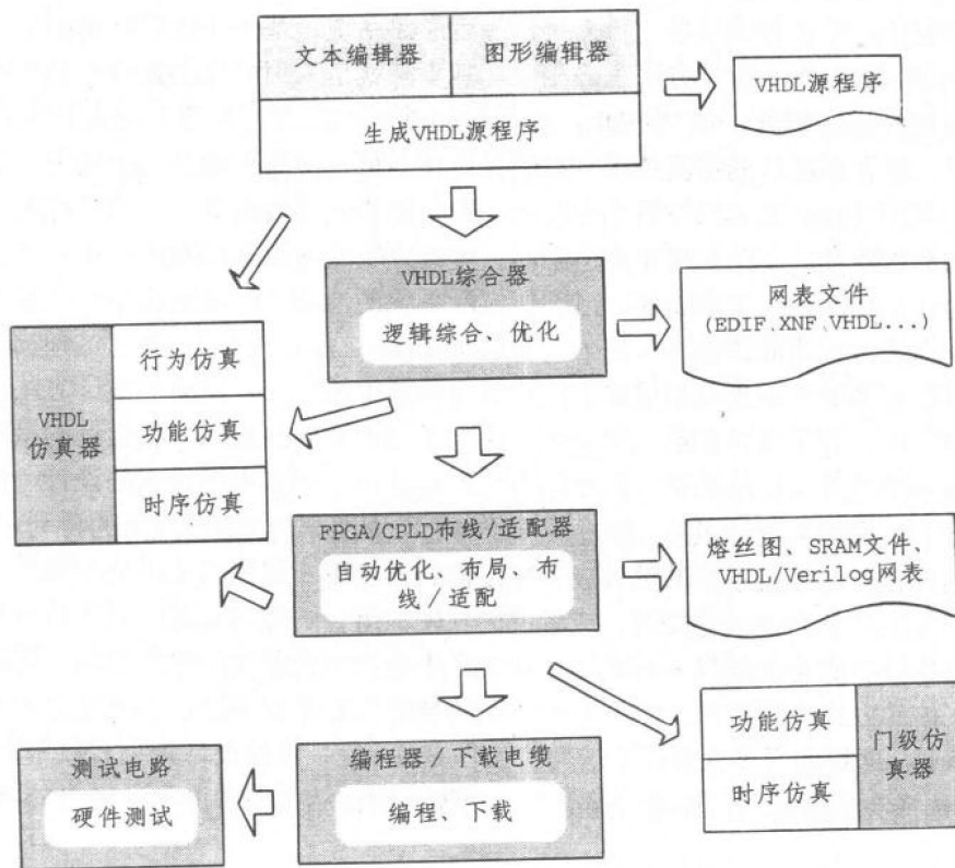
图 1-1 VHDL 工程设计流程图
