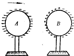
图1.1-8 静电感应
