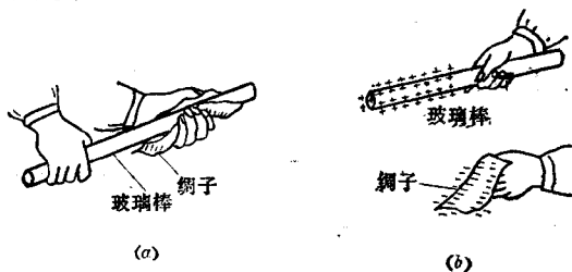
图 1.1-3 摩擦起电
