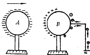
图1.1-9 感应起电
