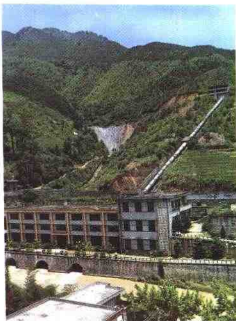
▲青印溪六级水电站
