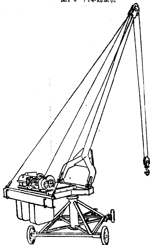
图1-8 小型起重机
