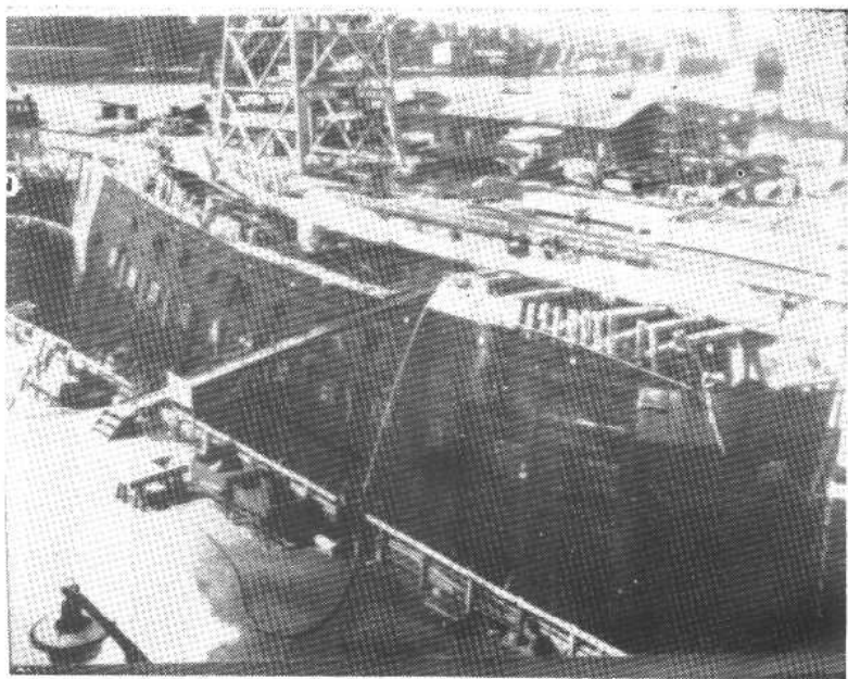
瑞典斯德哥尔摩的保护项目——十七世纪的战舰“瓦萨”号在修筑建筑物对它进行进一步的保护和陈列以前被放在为其特制的混凝土船坞里。
