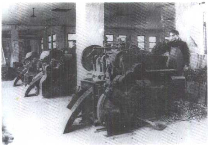
1954年9月1日，以私营利亚、一中、南明4家卷烟厂为基础组成公私合营贵阳卷烟厂。图为该厂当时的主要设备——制丝机。（贵州烟草公司袁通盛供稿）
