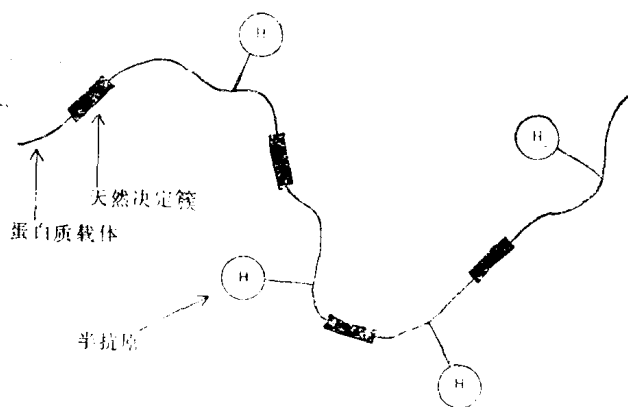
图3 半抗原-蛋白质结合物示意图。
