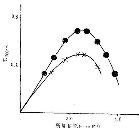
图2 在抗肌红蛋白血清中加入抹香鲸肌红蛋白(●—●)和原肌红蛋白(×—×)后形成的沉淀量。
