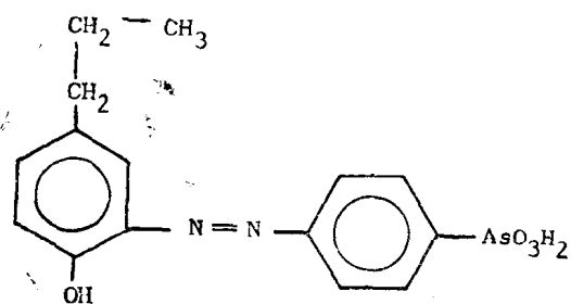
图5 (对-羟基苯)丙基-偶氮苯-对-砷酸 (RAN)。
