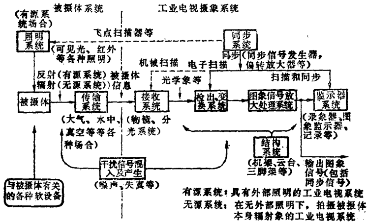
图 1.1 被摄体和摄象机组成图
