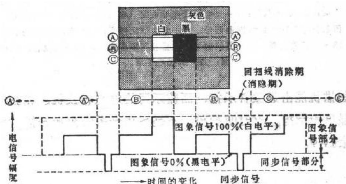
图1.4 复合图象信号
