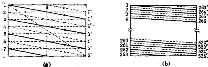
图1.8 隔行扫描
