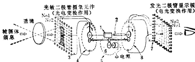
图1.3 使放大器和传输线合为一体的结构方案图
