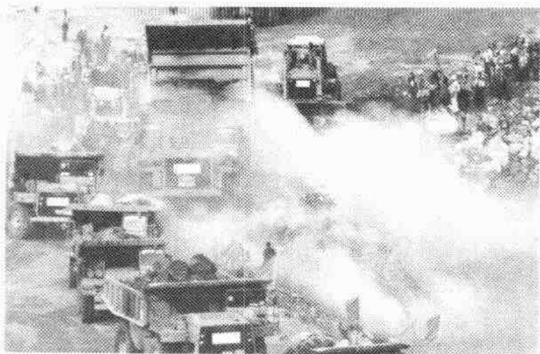
1997年11月8日,举世瞩目的长江三峡水利枢纽工程胜利实现大江截流。图为400多辆巨型装载车紧张有序地向围堰口抛投石料。
