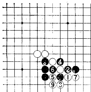
图 6 (黑 8 提劫=1 之左)
