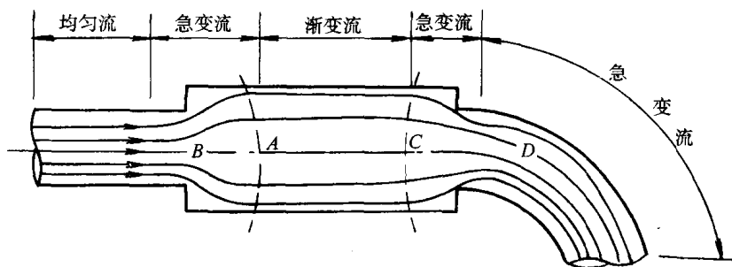
图 1-11 均匀流和非均匀流
