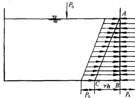
图 1-6 水池壁压强分布
