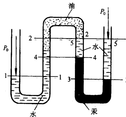
图 1-4 等压面与水平面
