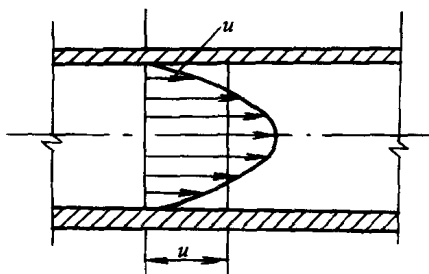
图 1-14 断面流速
