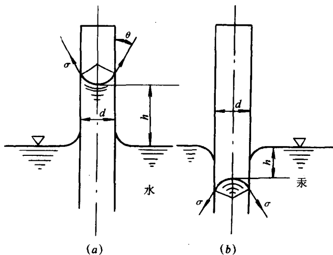
图 1-2 毛细管现象
