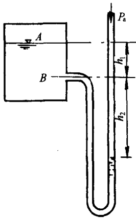
图 1-7 测压管
