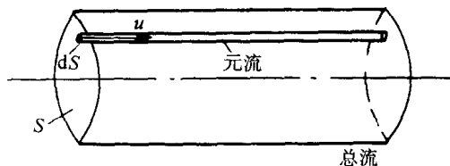
图 1-12 元流与总流
