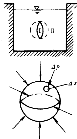
图 1-3 流体的静压强
