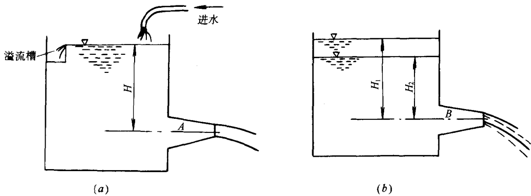
图 1-10 恒定与非恒定流动 (a) 恒定流动; (b) 非恒定流动
