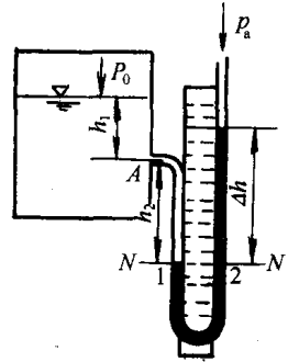
图 1-8 水银测压计
