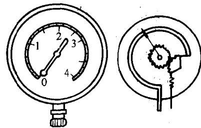
图 1-9 弹簧压力表
