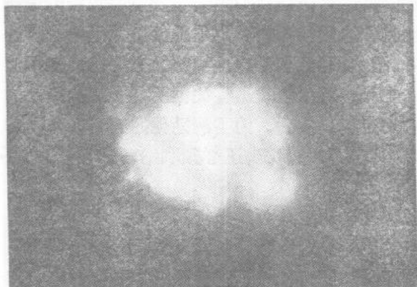
这是一张复制的照片，使它的底片曝光的只能是从铀盐发出的某些不可见的穿透辐射的结果，因为光不能照射到底板上。
