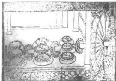
徐光启著《农政全书》插图“水转连磨”。
