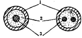
图 1-12 铠装热电偶断面 1—金属套管；2—绝缘材料；3—热电极
