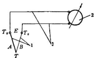
图 1-2 热电温度计组成
