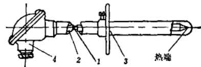
图 1-10 普通热电偶结构
