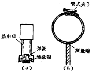
图 1-13 表面热电偶
