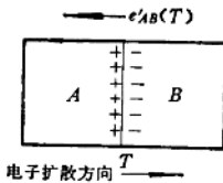
图 1-5 接触电动势
