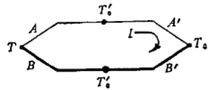
图 1-4 多个导体组成的热电偶回路
