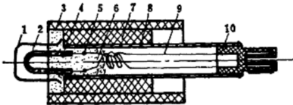
图 1-11 快速微型热电偶结构
