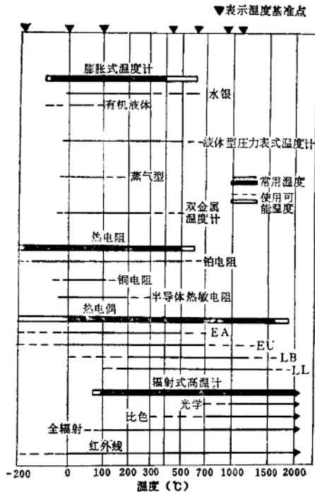
图 1-1 常用温度计及测量范围
