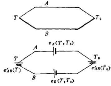
图 1-7 热电偶回路的总热电势
