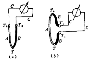
图 1-8 第三种导体 C 接入
