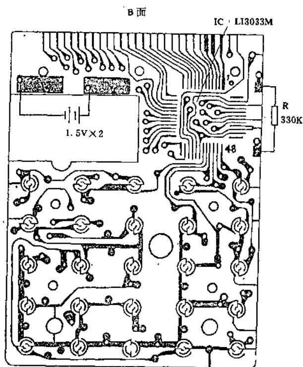
YX-087(KC-101B)印制板电路图
