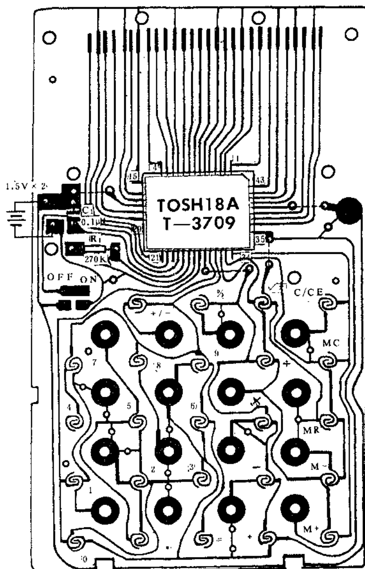
天鹅牌 KC-133型电子计算器 印制板电路及布线图
