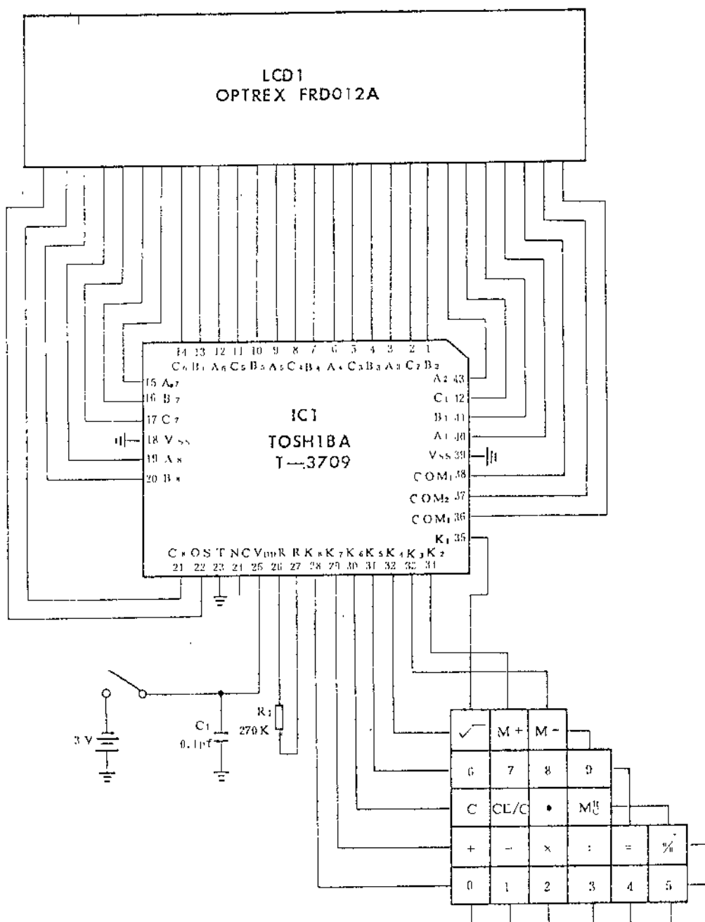
天鹅牌 KC-133型电子计算器电原理图
