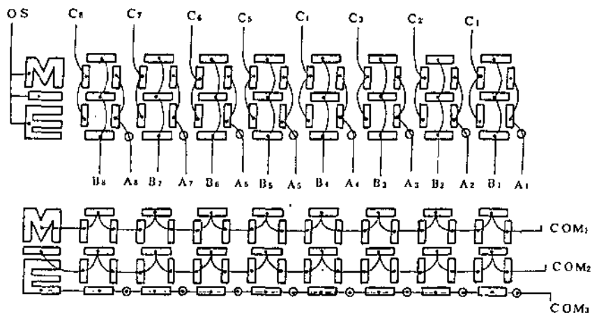
天鹅牌 KC-133型电子计 算器液晶显示引线图(FRD012A)
