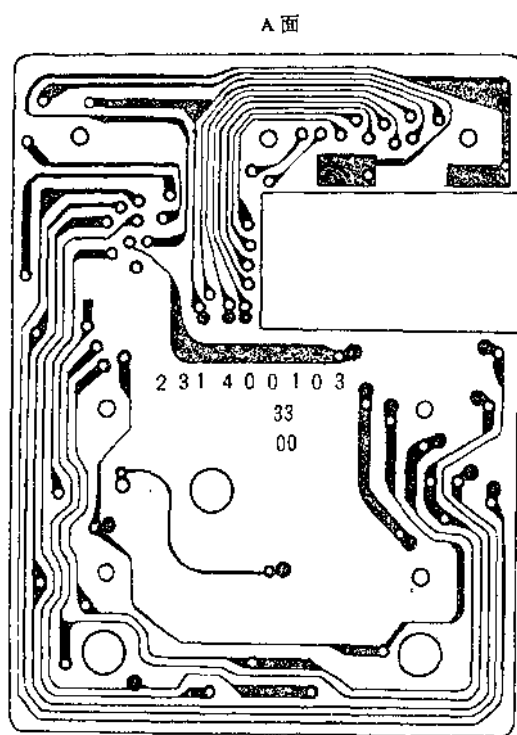
YX-087(KC-101B)印制板电路图
