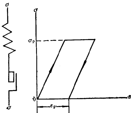
图 1-3 线性弹塑性介质
