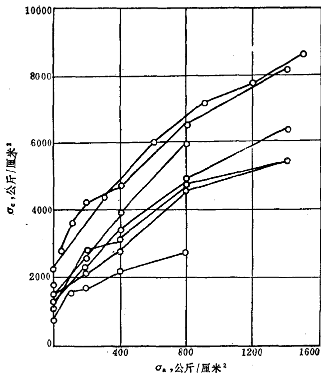
图 1-7 岩石三向压缩强度
