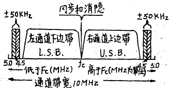
图3 立体TV发射机的频率分配
