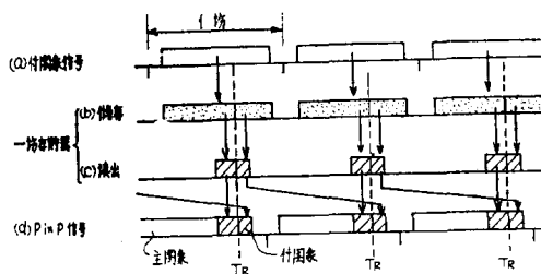
图10 一场存储系统的定时曲线图(1)
