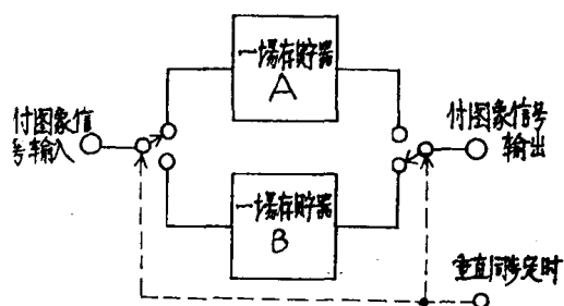
图7 二场存储系统的存储器结构
