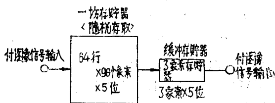
图9 一场存储系统的存储器方框图
