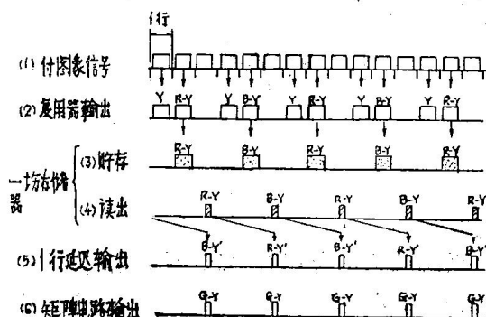
图6 色处理定时曲线图
