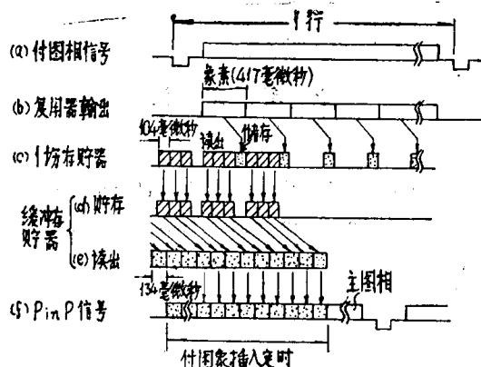
图11 一场存储系统的定时曲线图(2)
