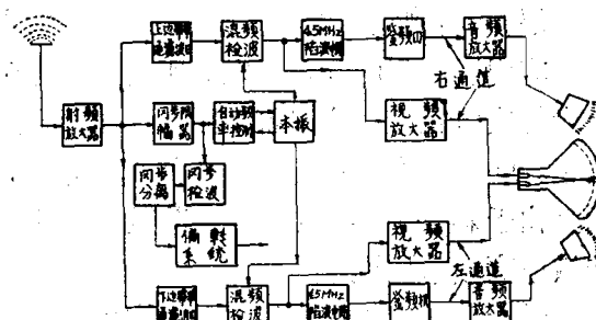
图4 立体电视接收机方框图
