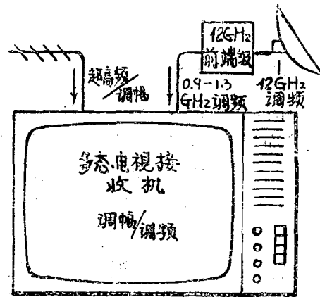
图3 能接收0.9—1.3千兆赫间的调频信号多态电视接收机，它是家用卫星接收机中最感兴趣的结构之一。
