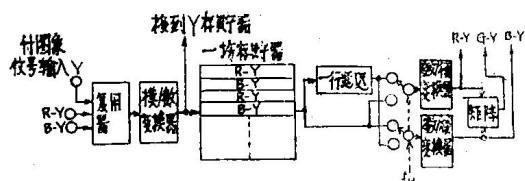
图5 色处理方块图
