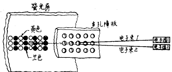
图1 被改进了的立体显象管部分
