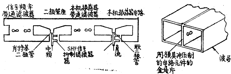
图5 日本广播协会为试验性的低成本卫星接收机研制的平面电路12千兆变换器详图,实质上它是具有冲出来以形成电路元件的金属片。实验元件具有要求的噪声指数4.5分贝,变频损耗3.4分贝。
