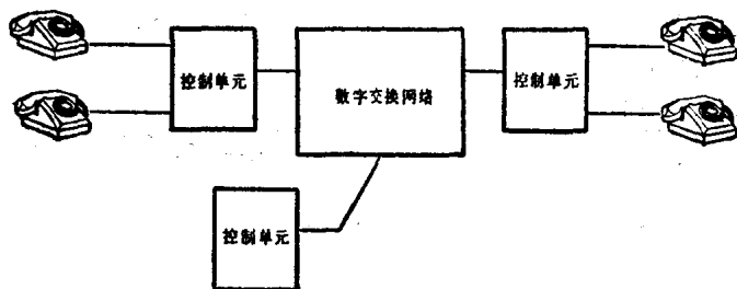
图1-1 S1240简化的系统结构
