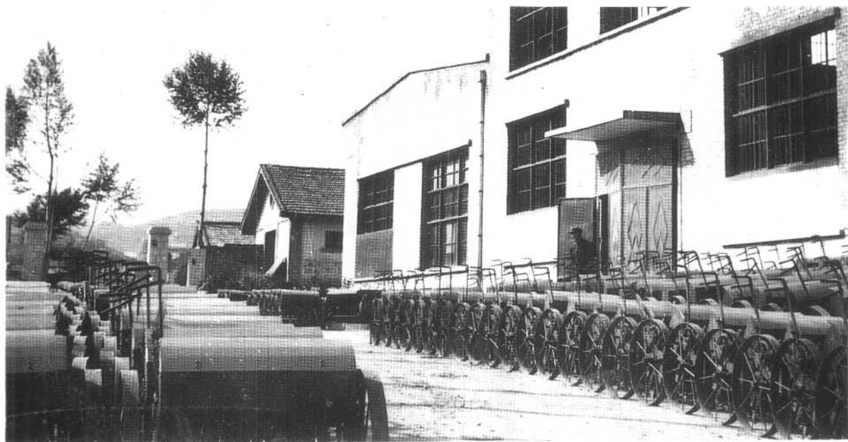
县农业机械厂生产的条播机
