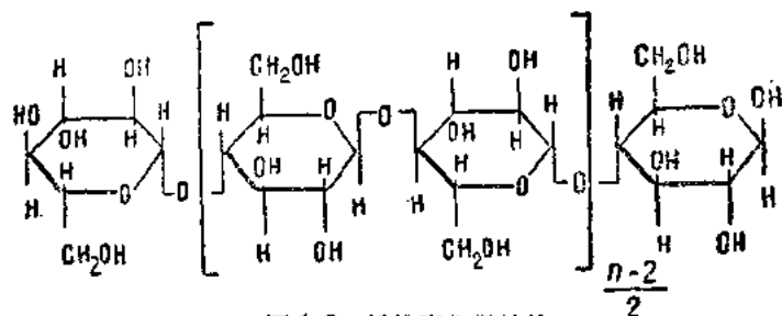
图 1-2 纤维素化学结构
