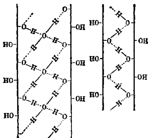
图 1-3 纤维素的氢键结合示意图
