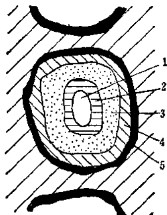
图 1-1 植物细胞壁结构 断面示意图
